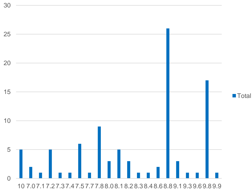
CVE par score CVSS
