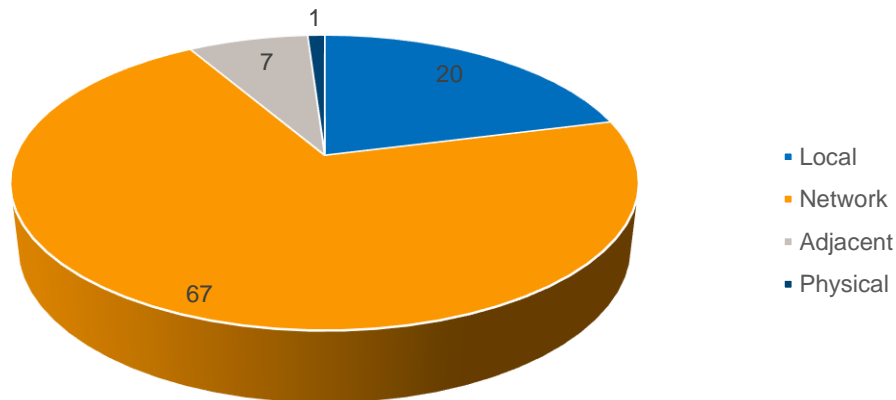
CVE par type de vecteur d'attaque
