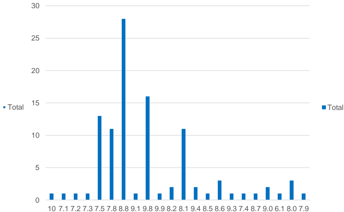
CVE par score CVSS
