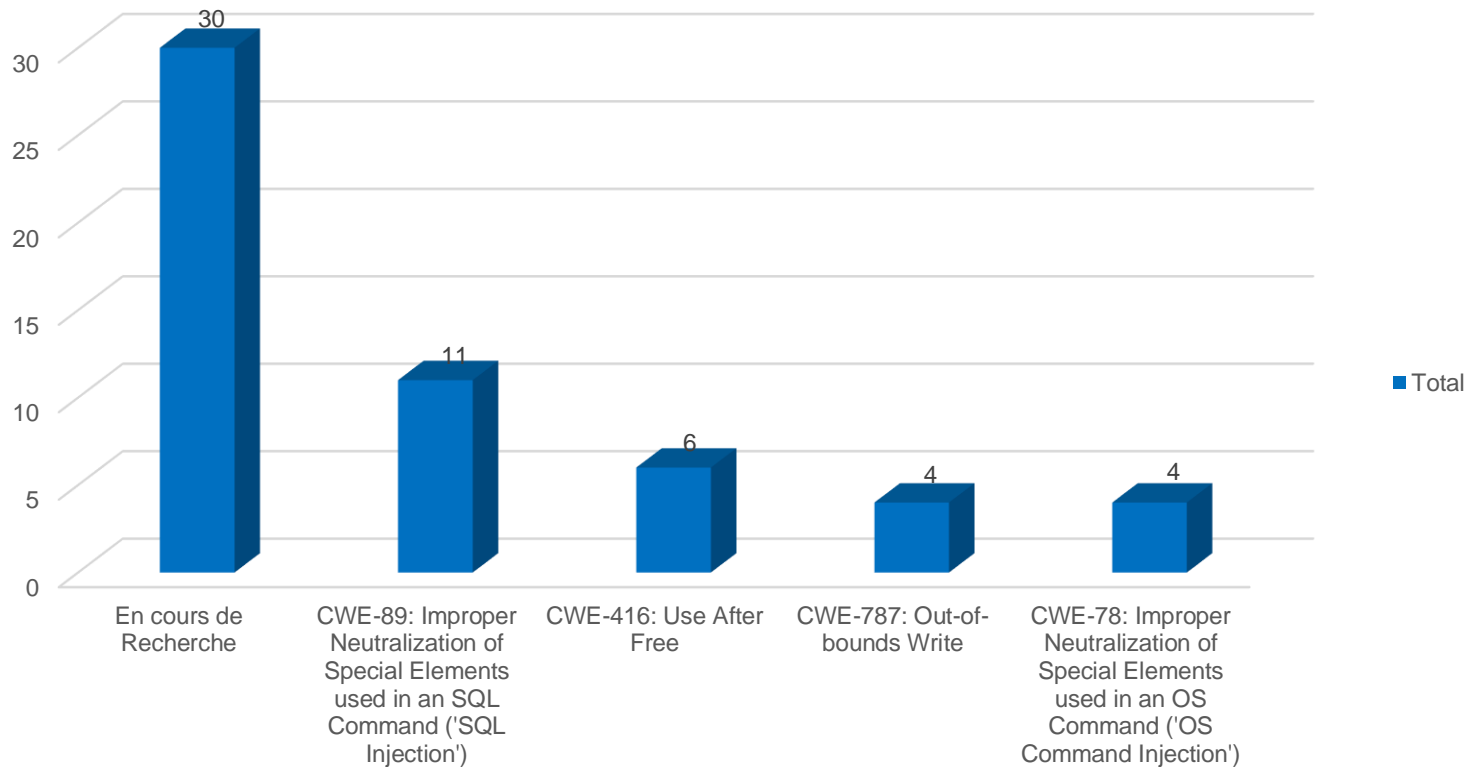
Nombre de CVE par CWE
